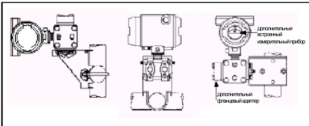
Рисунок 9 – Примеры типичных положений монтажа
