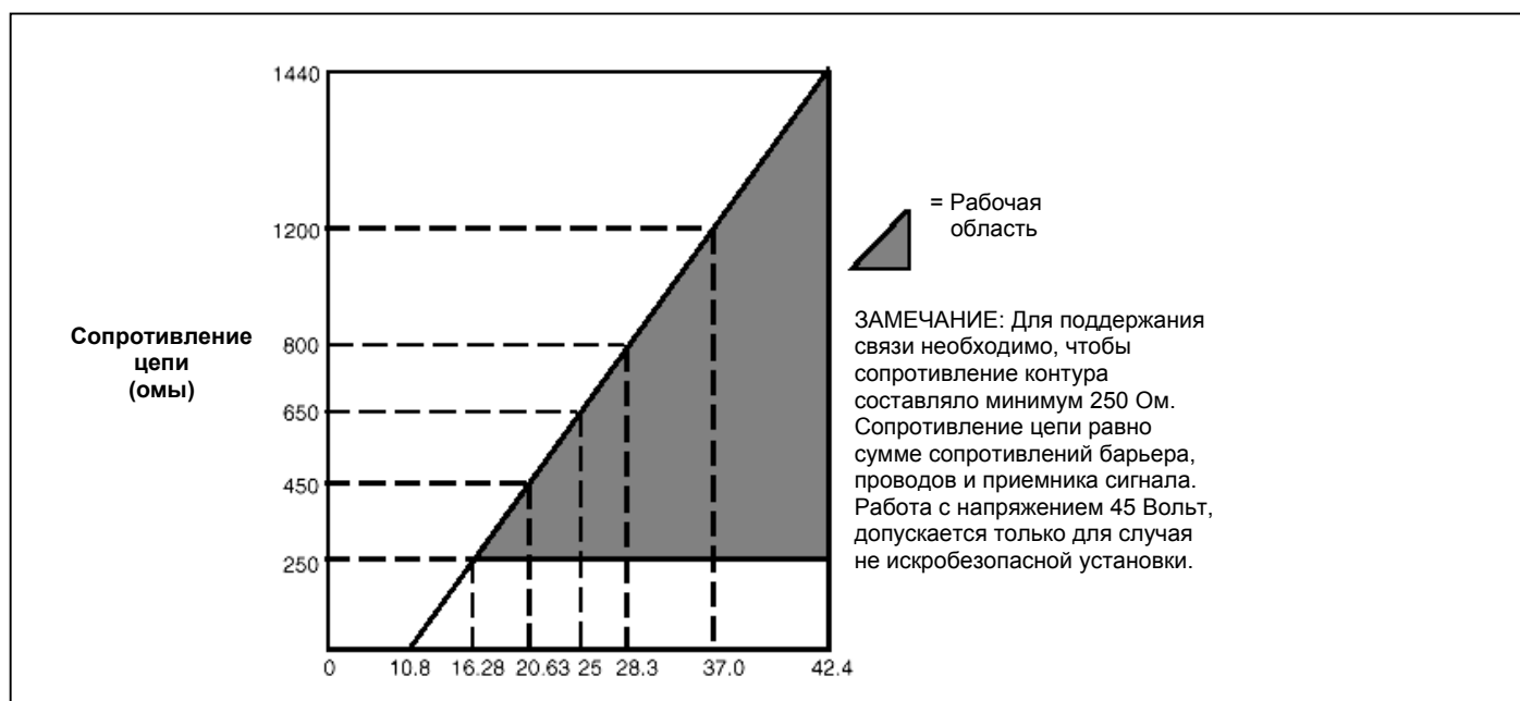
Рисунок 7 - График подаваемого напряжения и сопротивления цепи
