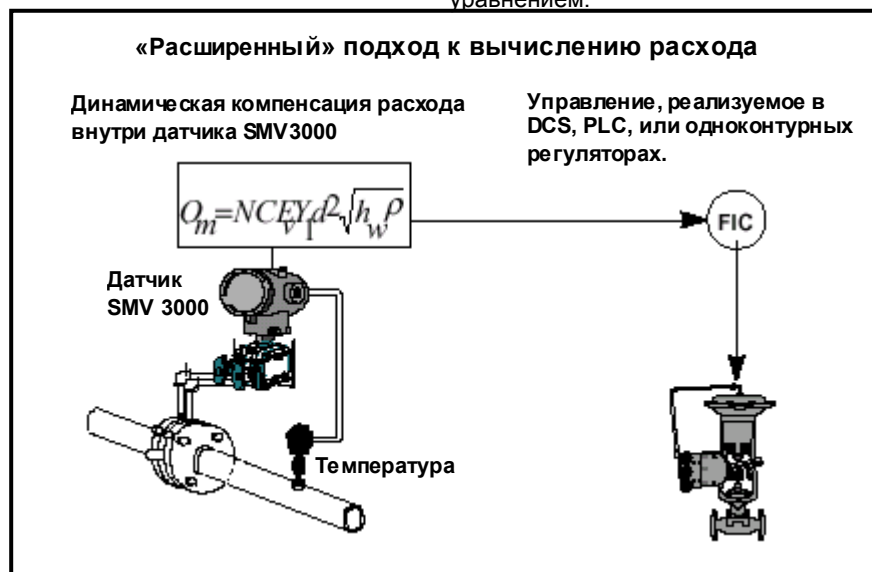
Рисунок 3 —Компенсация расхода с использованием “Расширенного” подхода
