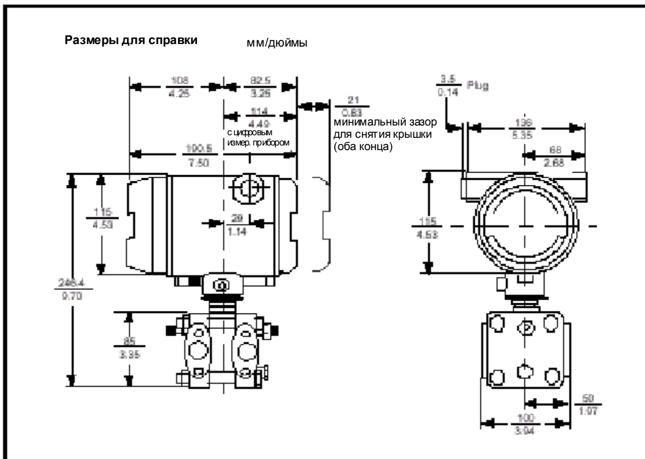
Рисунок 8 - Приблизительные монтажные размеры только для справки.
