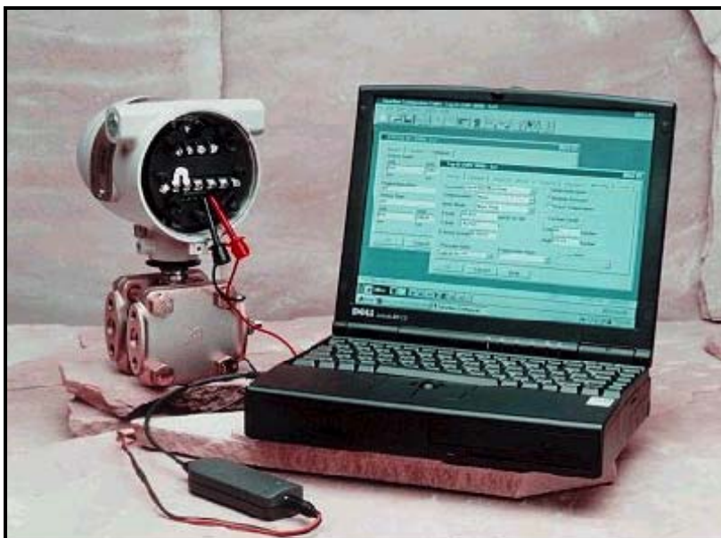
Рисунок 1 —Интеллектуальный многопараметрический датчик расхода SMV 3000 с интеллектуальными средствами конфигурации SCT 3000. Датчик SMV 3000 измеряет дифференциальное давление, статическое давление, температуру технологического процесса и на основании этих измерений динамически вычисляет массовый и объемный расход.
