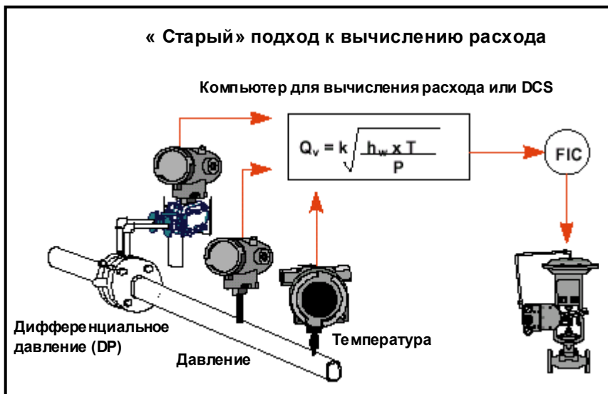
Рисунок 2 —Компенсация расхода с использованием “Старого” подхода
